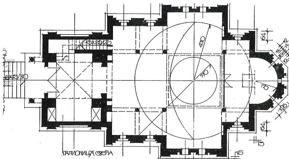
Основа (план) будуће цркве у Белошевцу.
